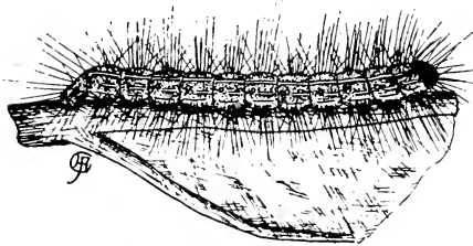
Fig. 483. Malacosoma americana Fab.
